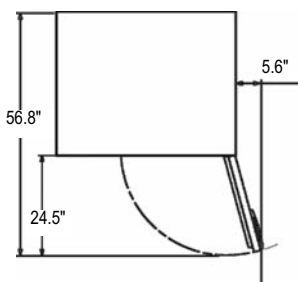
HUR40A (DOOR SWING)
